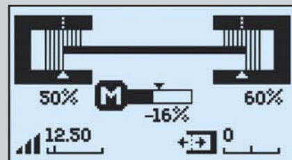
Affichage graphique du masquage de palpeur, de la position du moto-vérin, du gain et de la consigne
