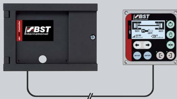
Amplificatore ekr 500 con tastiera remota
